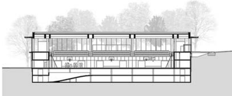
Coupe transversale
